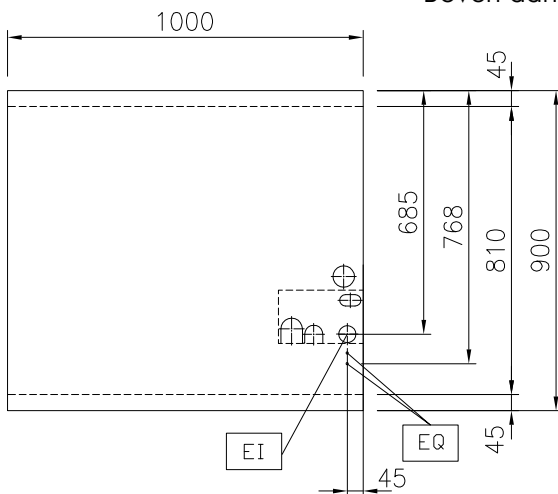
Boven aanzicht
